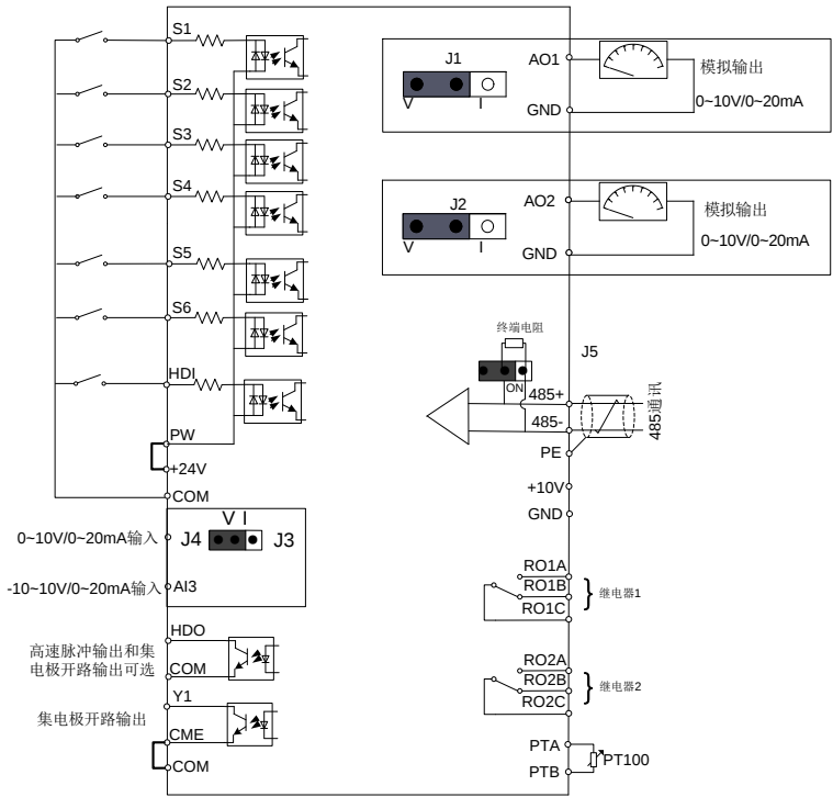
图 3-4 三相 18.5kW（含）以上机型控制端子接线
