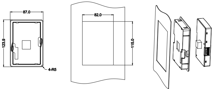
2.2~15kW键盘安装架（选配）图
