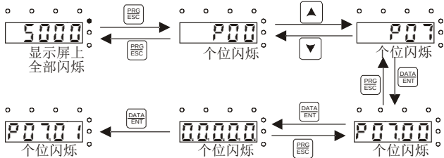
图 4-4 设定密码
