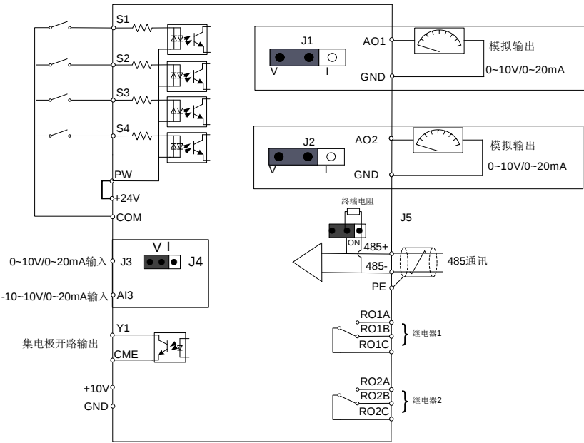
图 3-2 单相机型控制端子接线
