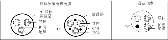
图 B-1 对称屏蔽机电缆
