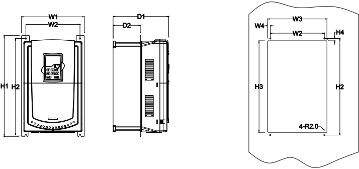
图 A-9 37~110kW 法兰安装
