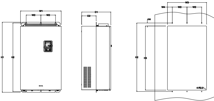
图 A-10 132~200kW 法兰安装
