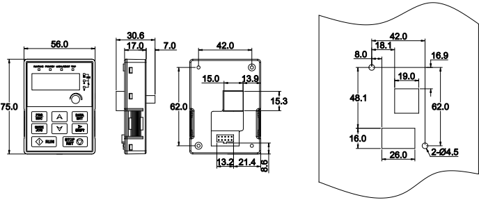
单相220V外引键盘结构图
