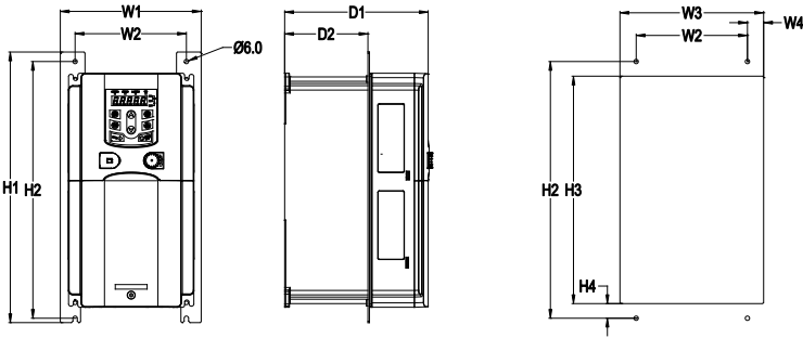
图 A-7 2.2~15kW 法兰安装
