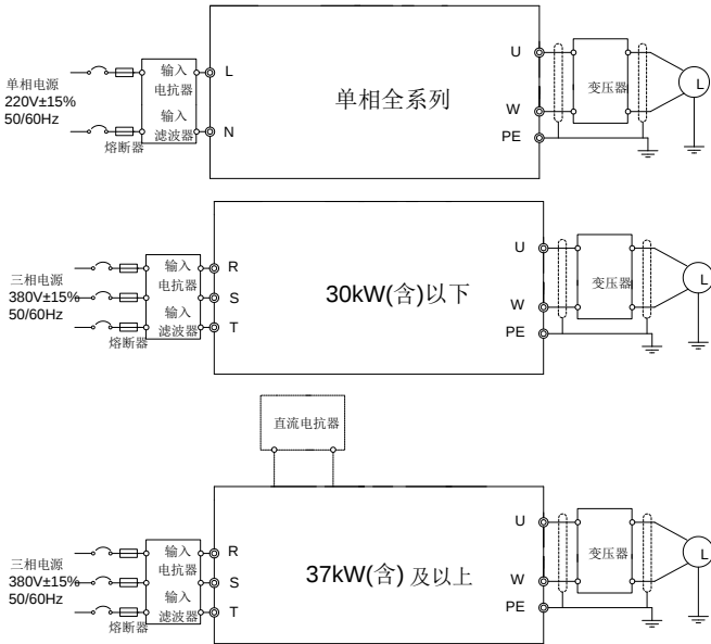
图 3-1 主回路接线
