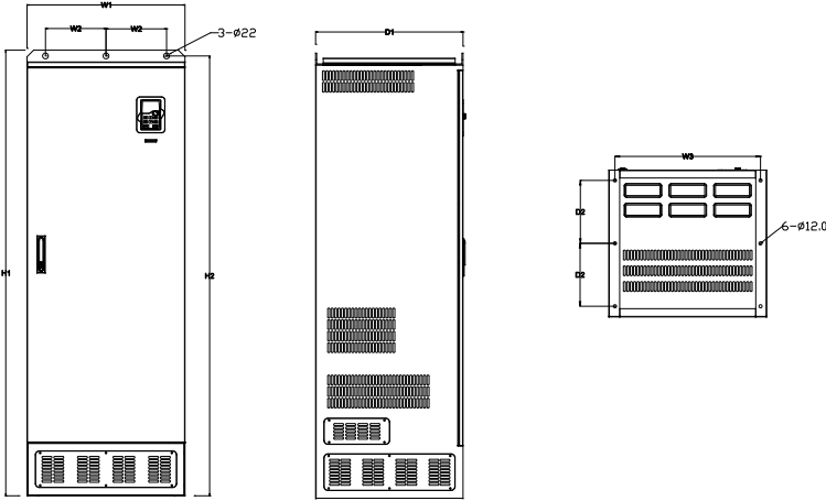
图 A-12 350~500kW 落地安装
