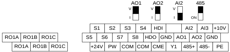
图 3-6 15kW（含）以下控制端子
